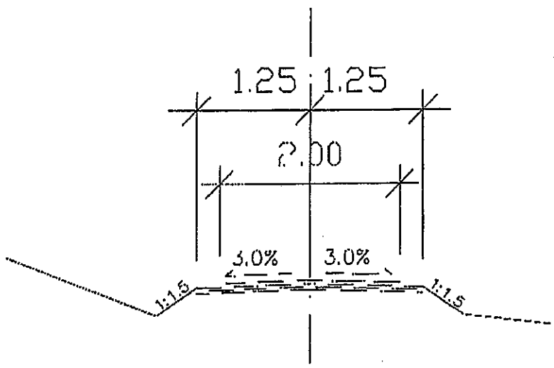
.verrsnitt gangveg
