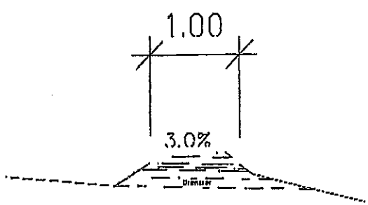
Tverrsnitt gangsti
